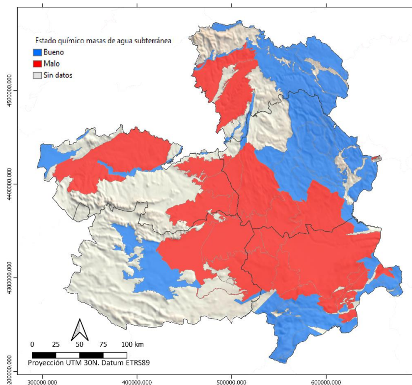
Estado químico de las masas de agua subterránea de Castilla – La Mancha 2015-2021. Elaboración propia. Fuente: MITERD
