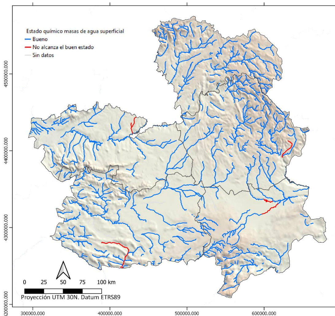
Estado químico de las aguas superficiales de Castilla – La Mancha 2015-2021. Elaboración propia. Fuente: MITERD
