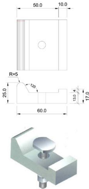
TACO DE ALUMINIO (cotas en mm)
